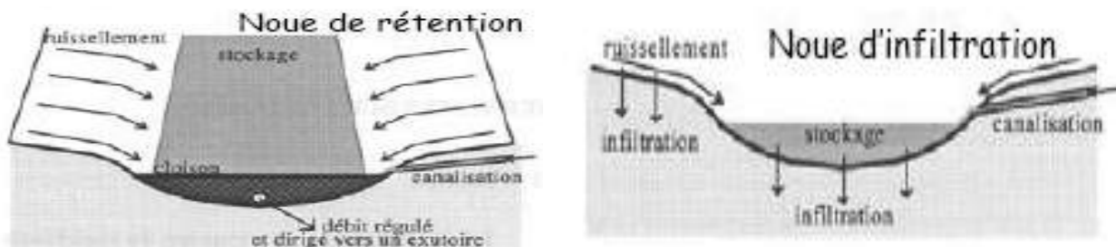
Figure 4 : Schéma de principe d'une noue
